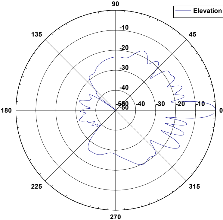
26 6008 XP XP MIMO Elevation Pattern
