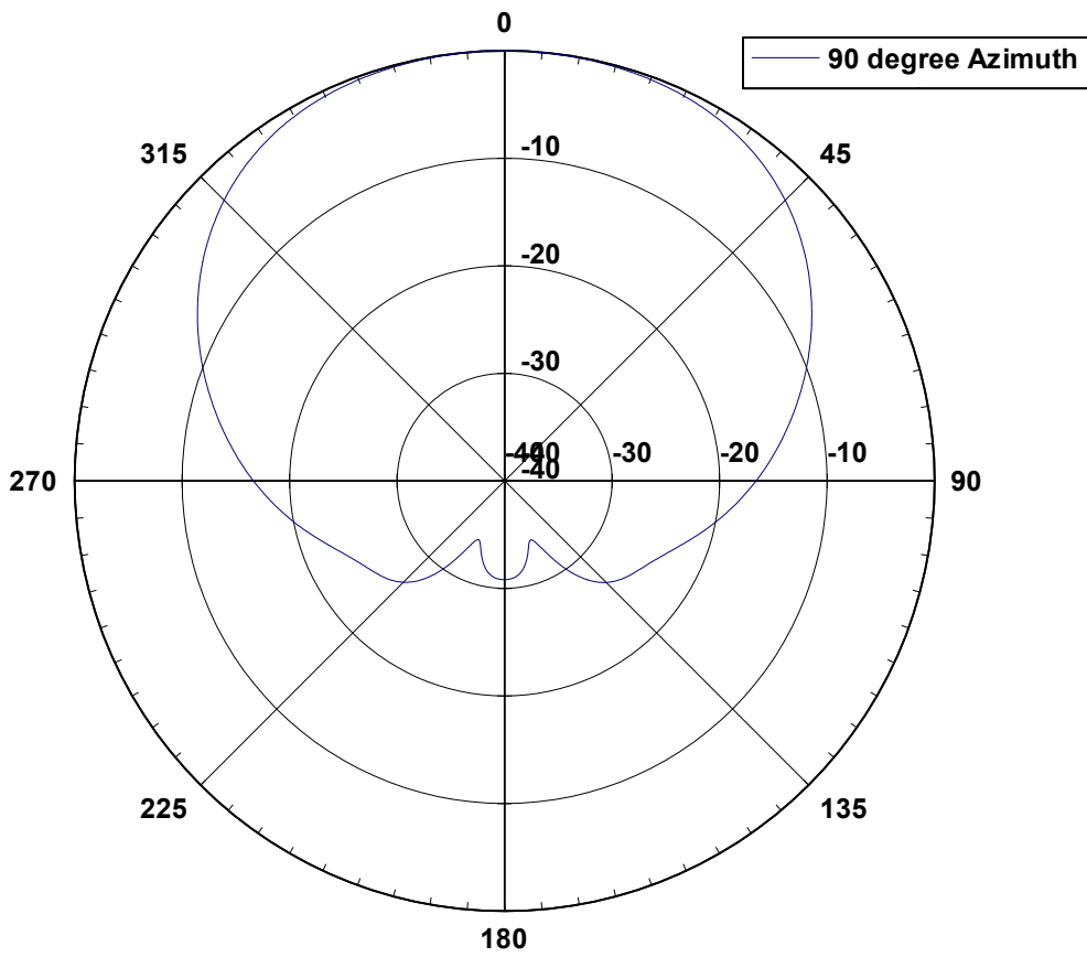
24 9010H Elevation Pattern
