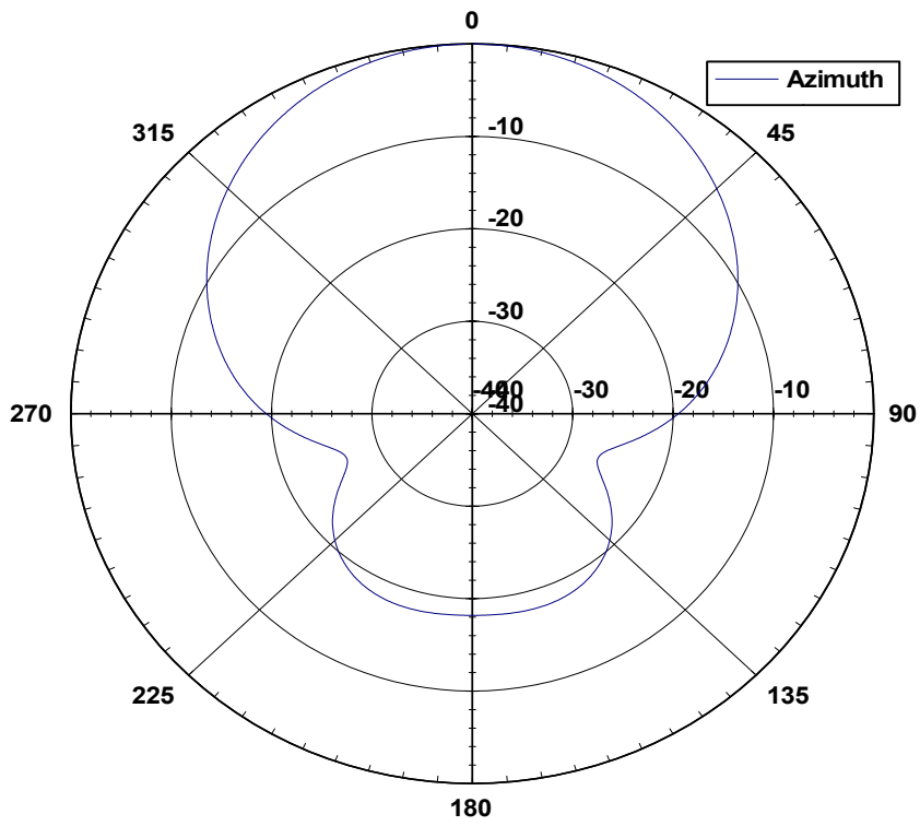
24 8080 OB Azimuth Pattern
