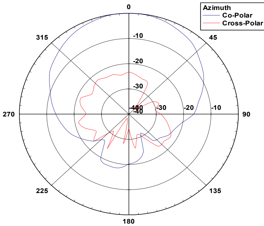
24 8040 OB Azimuth Pattern
