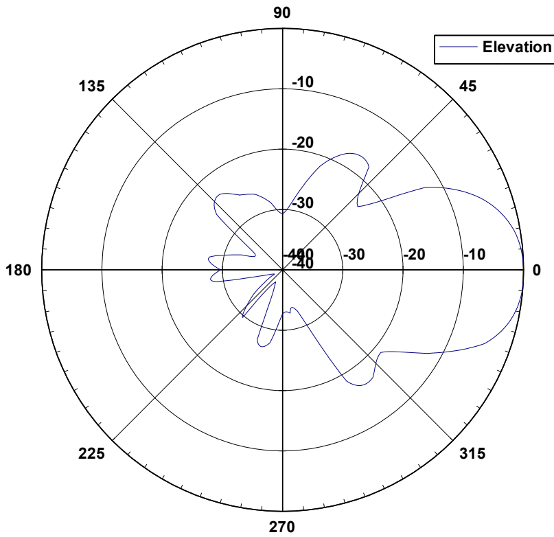
24 8040 OB Elevation Pattern
